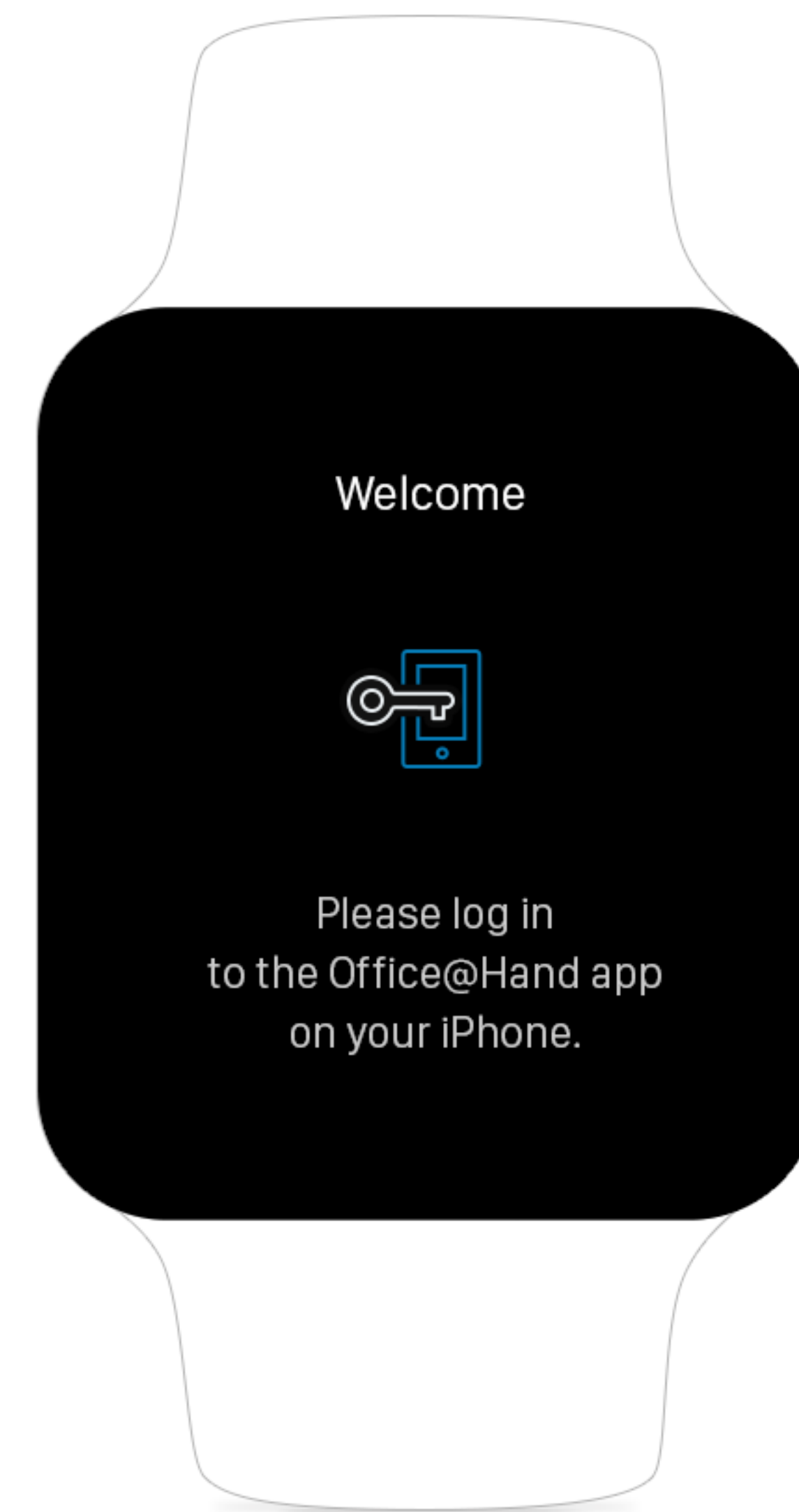
3. Un-login case
