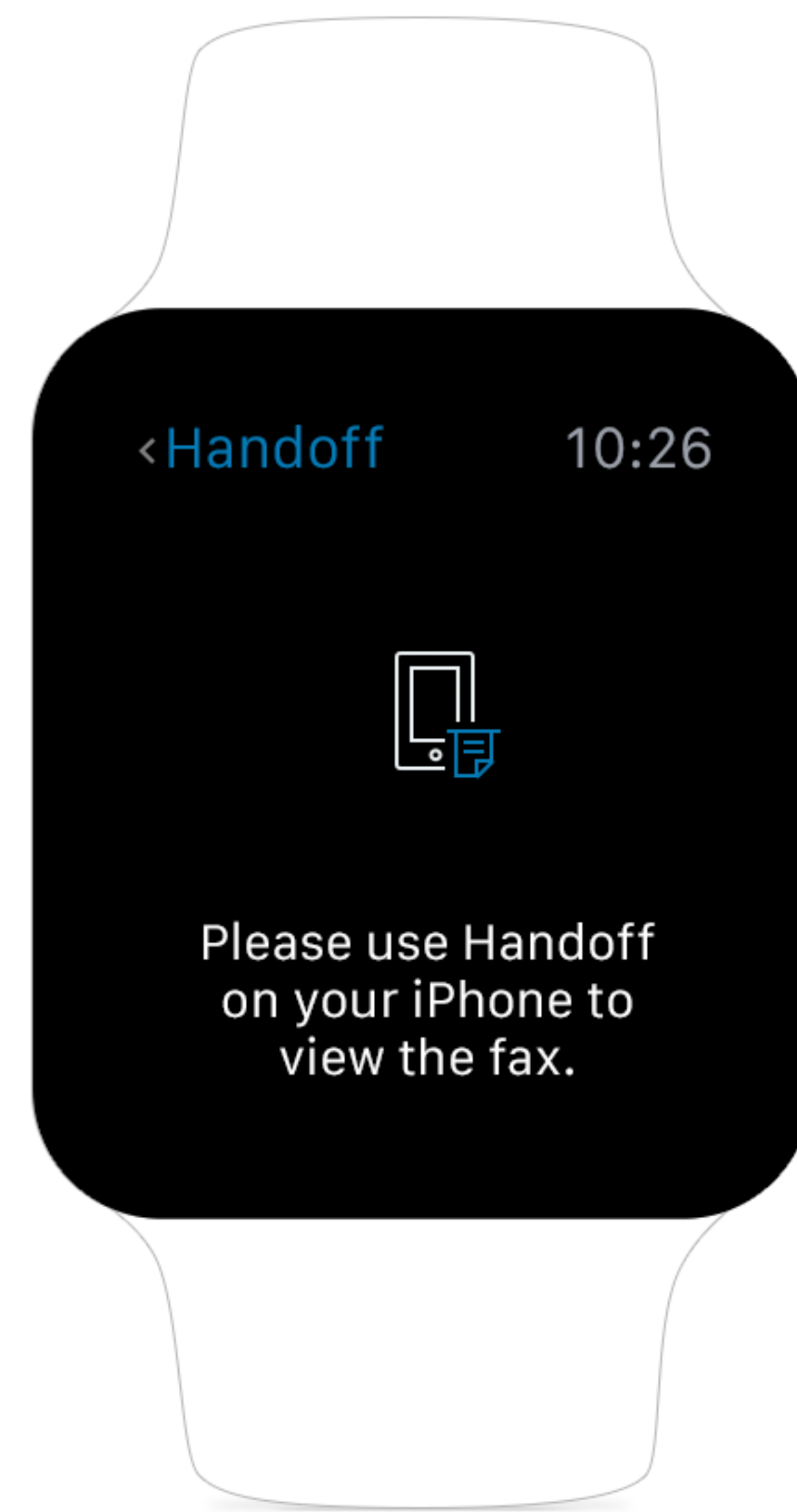
2. Fax
